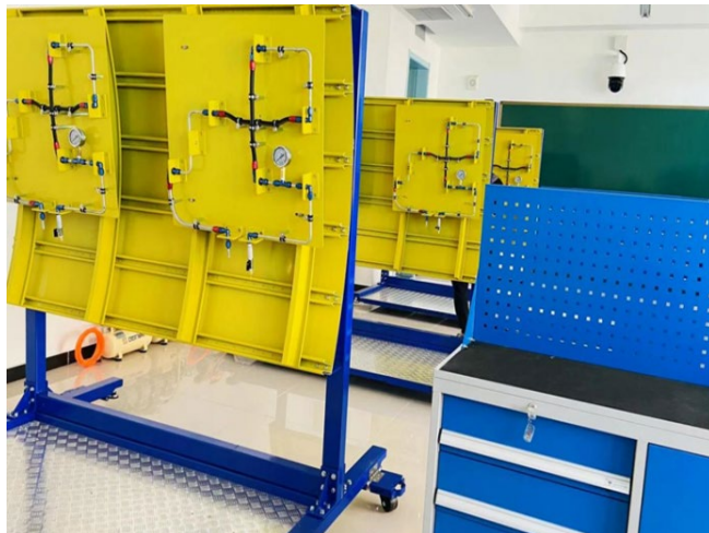
图 77：校企共建飞机维修专业实训室
